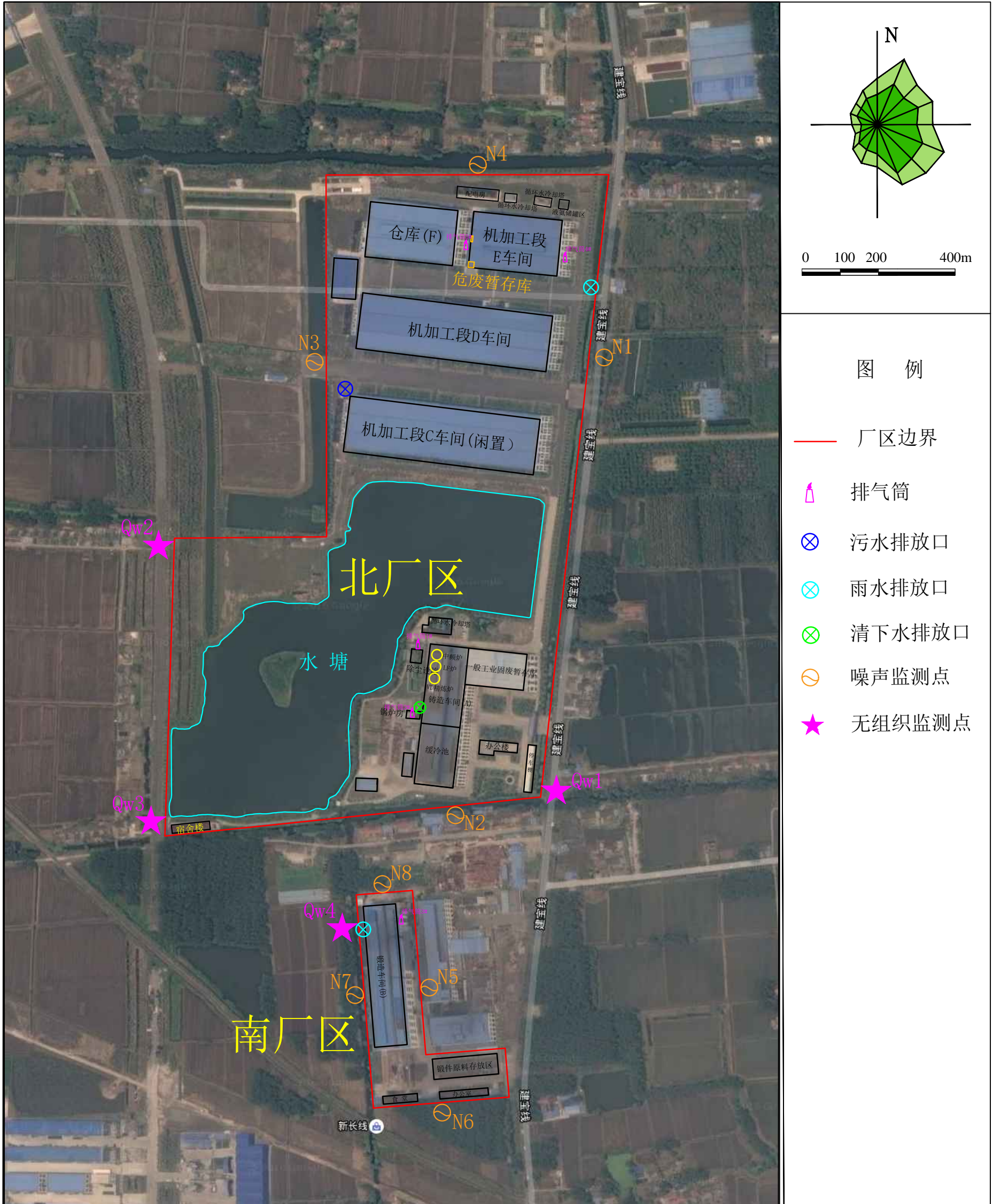
图3.1-2 项目平面布置图（含验收监测位点）
